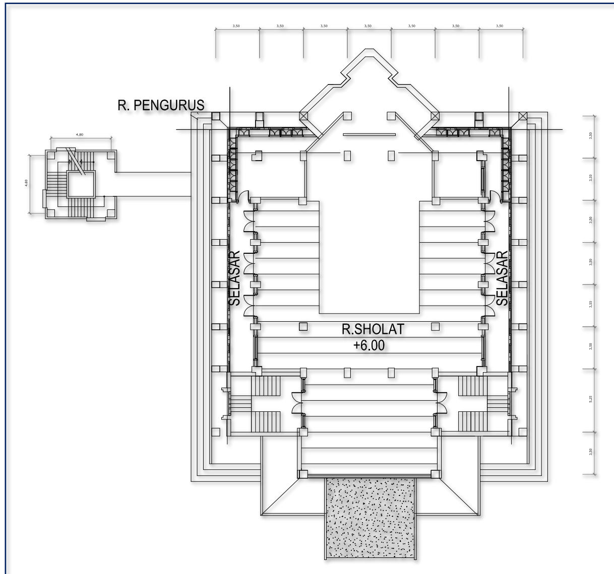
DENAH LANTAI ATAS MASJID SMA NEGERI 1
